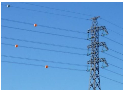
Bsp.: Kugelmarker montiert an Freileitung
